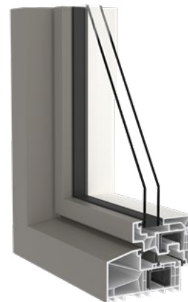
Cadre épuré avec ouvrant Fino en retrait
